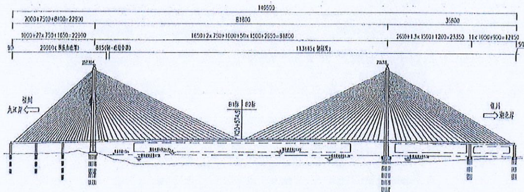
图 1.1 九江长江公路大桥主桥(斜拉桥)布置图
